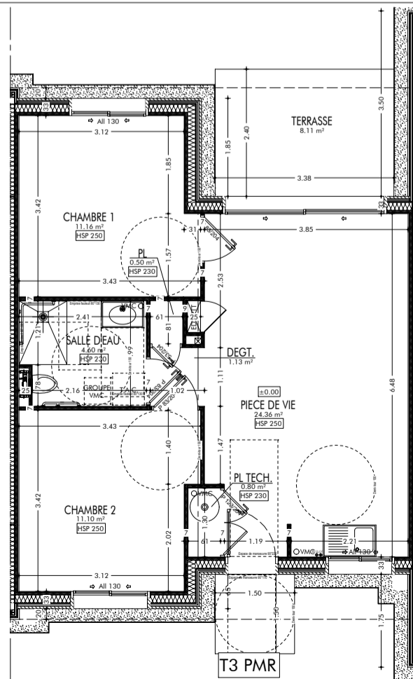
REZ-DE-CHAUSSEE
