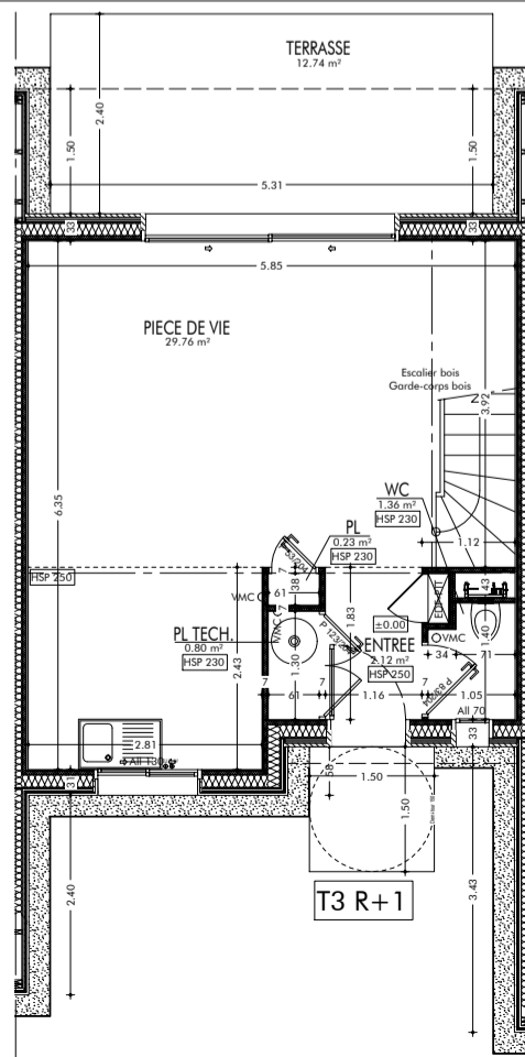
REZ-DE-CHAUSSEE
