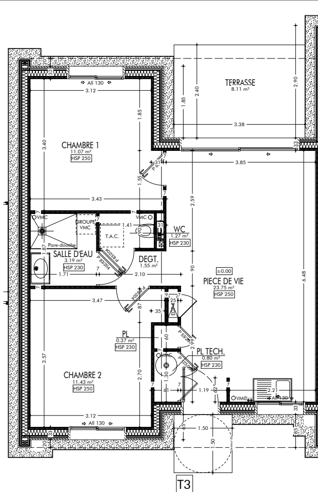
REZ-DE-CHAUSSEE
