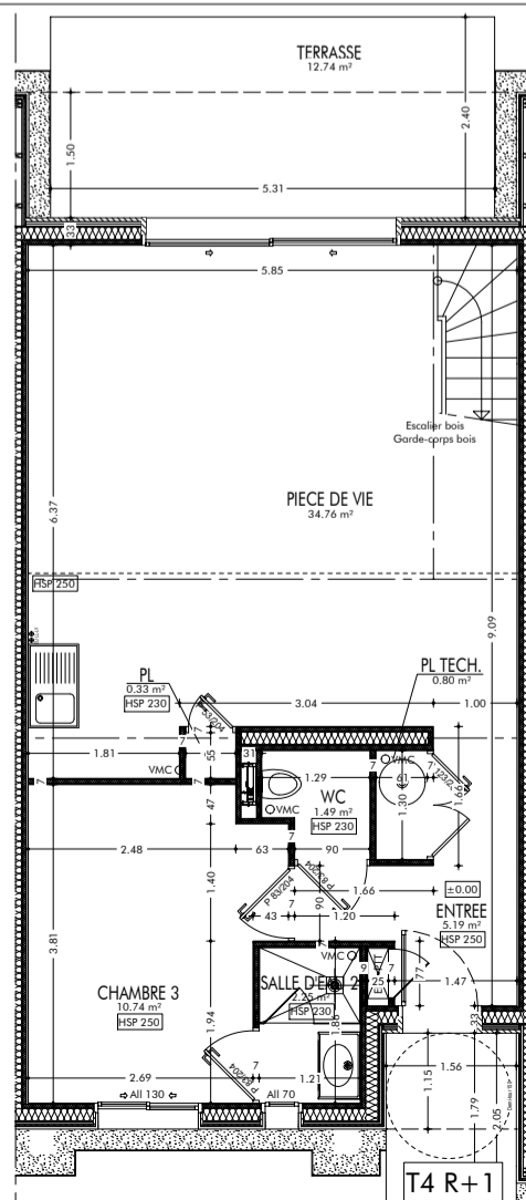
REZ-DE-CHAUSSEE
