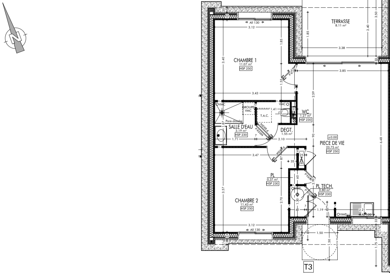
REZ-DE-CHAUSSEE
