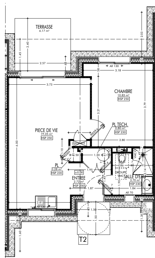
REZ-DE-CHAUSSEE
