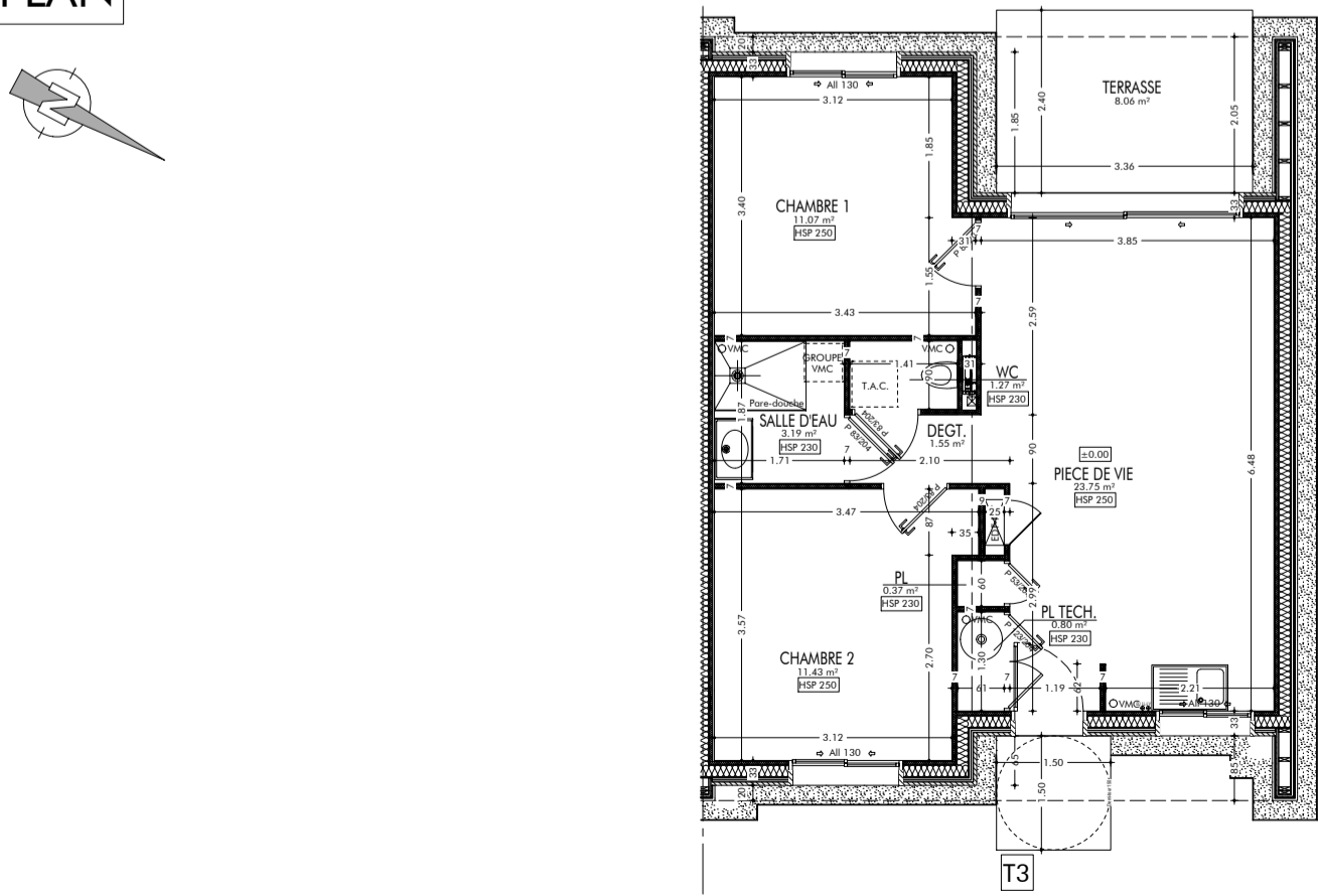
REZ-DE-CHAUSSEE
